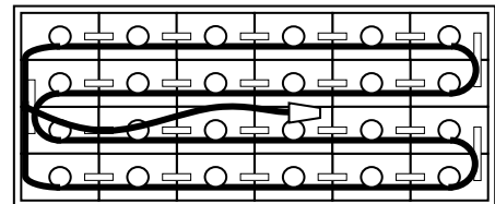
Voorbeeld opstelling BFSIII
